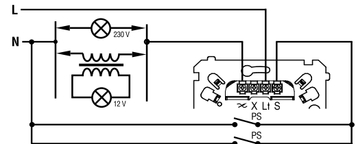
Рис. 5. Подключение к электрической сети с дополнительной кнопкой (PS) со стороны «нуля»
