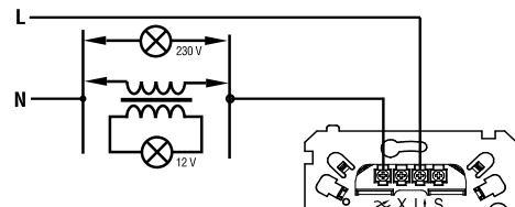
Рис 2. Подключение к стандартной электрической сети
