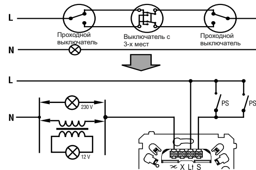
Рис. 4. Подключение к электрической сети с дополнительной кнопкой (PS) со стороны фазы
